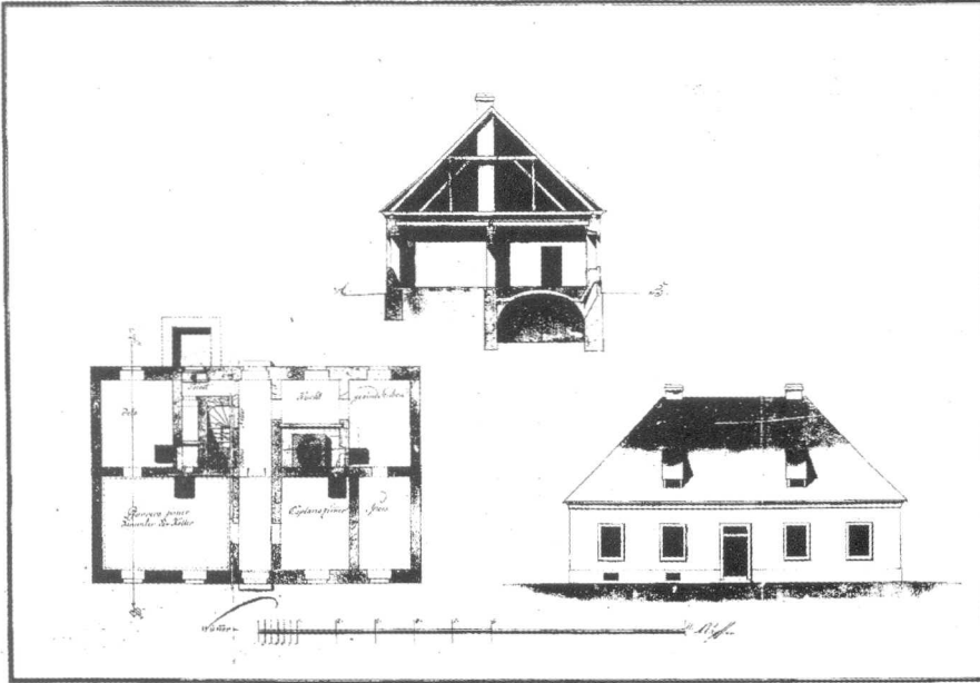
4. A Budaörsi paplak tervrajza (No 511/7)
