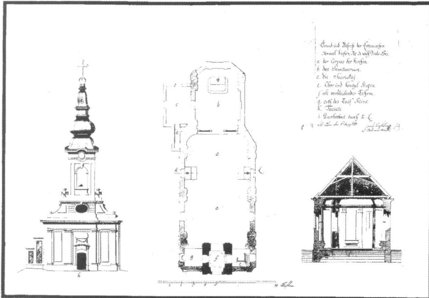
3. A budaörsi (harmadik) római katolikus templom alap- és homlokzati tervrajza (No 216/4)
