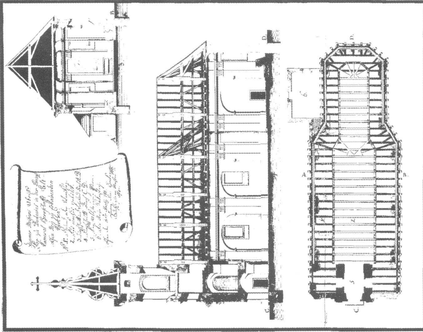
2. A királyi kamarai Óbudai uradalomban, Budaörsön újonnan építendő templom ácsmesterei alaprajza (No 197/9)
