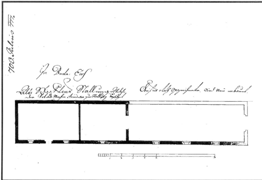
21. A budaörsi régi juhakol alaprajza (No 157)
